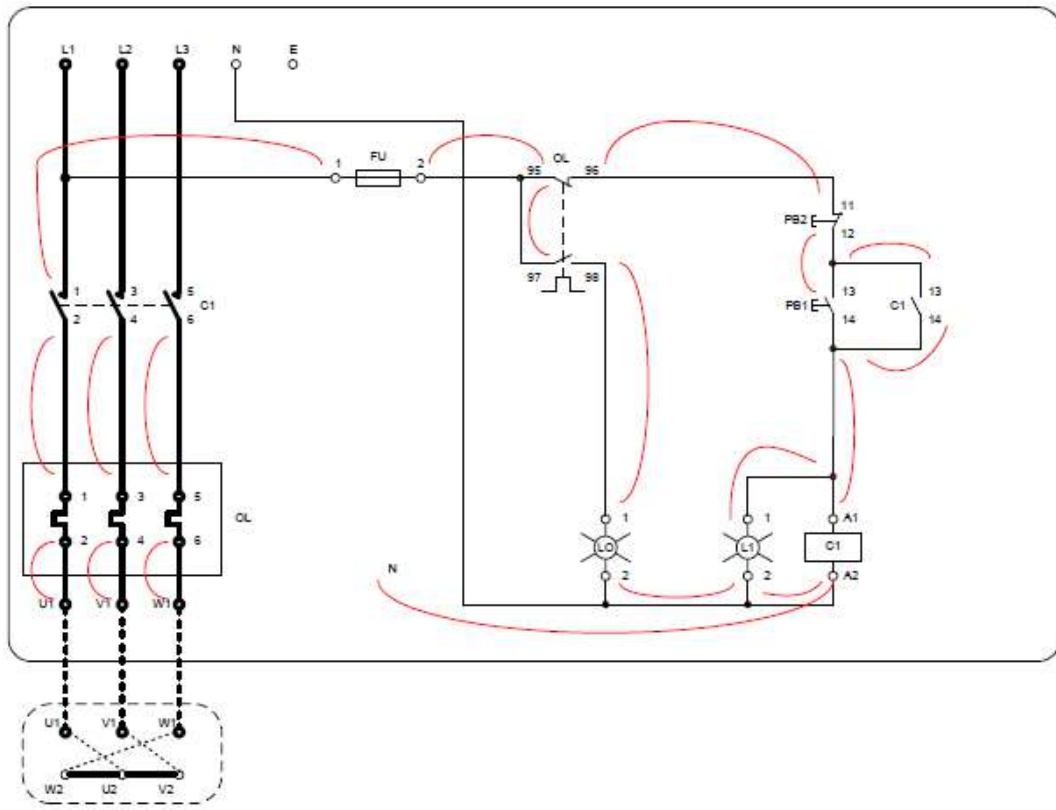
佈線圖
