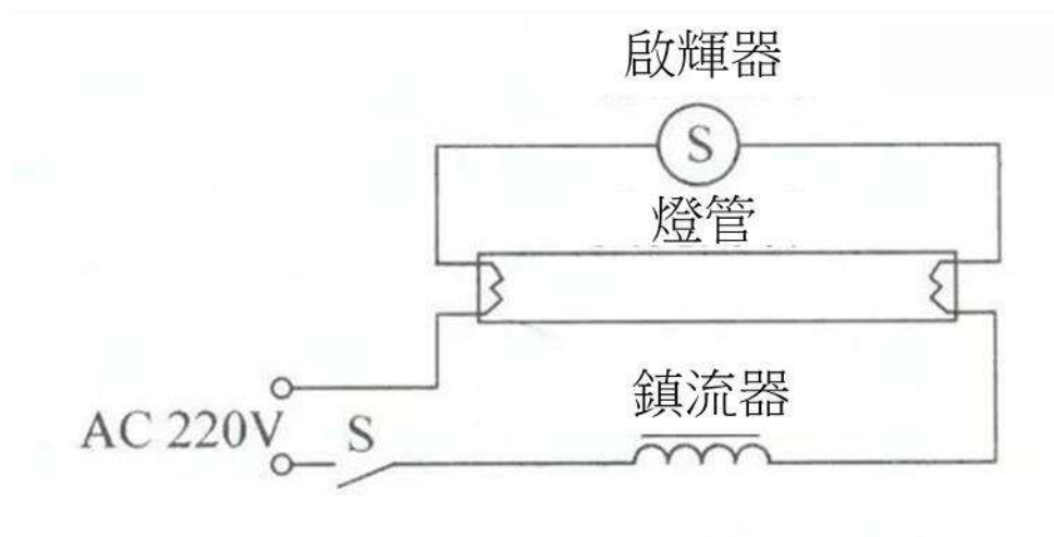
照明電路
